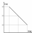
Wykres maksymalnych obciążeń masztu przy podniesieniu wózków powyżej 2 m, obciążenie maleje zgodnie z wykresem
